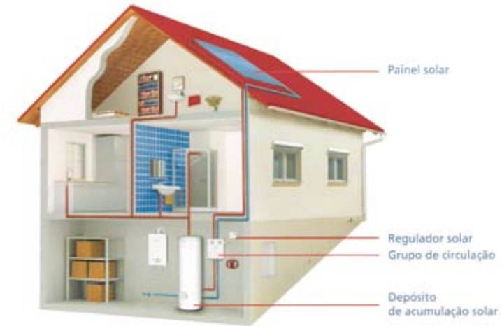
Instalação de 54 colectores solares térmicos para aquecimento de águas sanitárias IPSS em Setúbal
